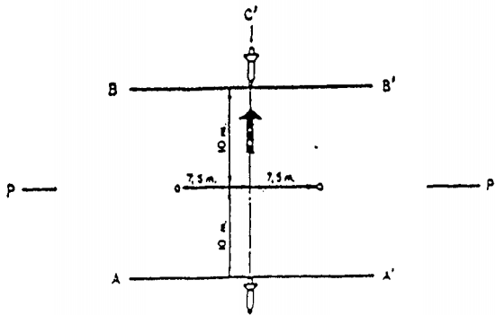
Figura 1: Posiciones de ensayo de las moto cicletas en marcha.
